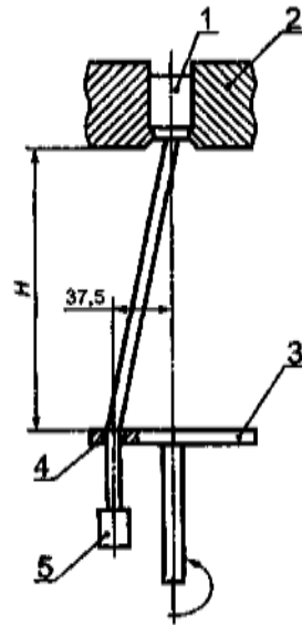
1 — зажим; 2 — подставка; 3 — плата; 4 — втулка; 5 — груз Рисунок 1 — Испытательная установка
