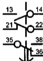
Три контактных элемента
